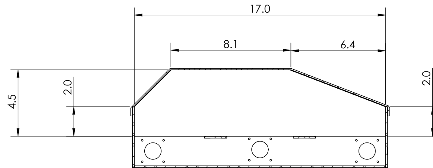
SECTION A-A
